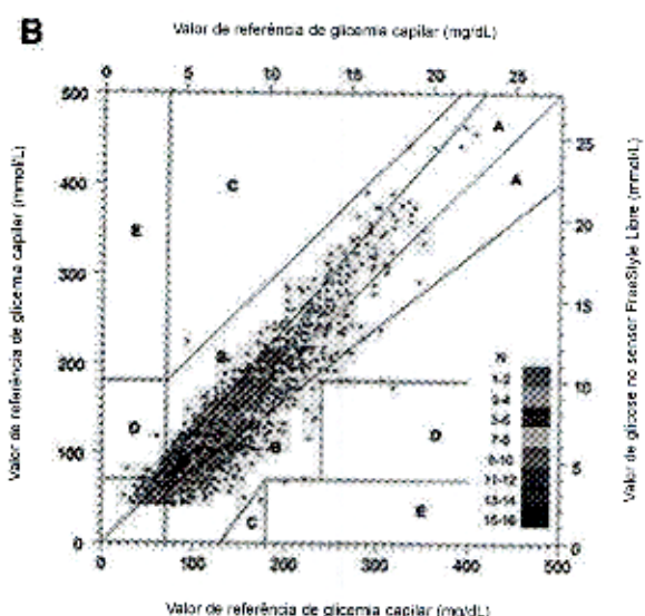
FIGURA 1. Análise de grade de erro de consenso (A) e de Clarke (B), comparando resultados de sensor FreeStyle Libre a resultados de glicemia capilar. BG, glicemia
